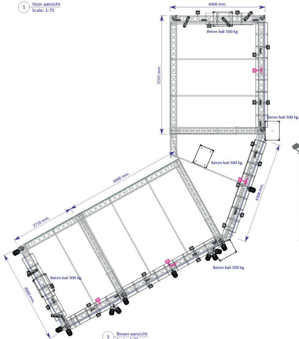
3 Boven aanzicht Scale: 1:75
